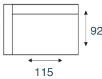
1 zits met eiland L|R 17774/17775 HR
